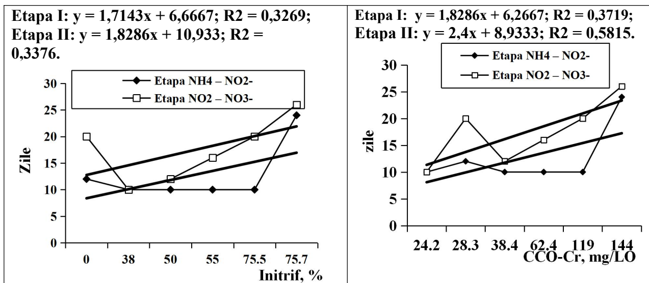
Figura 23. Corelarea duratei (zilelor) etapelor procesului de nitrificare cu valoarea Indicelui de nitrificare a apei.
